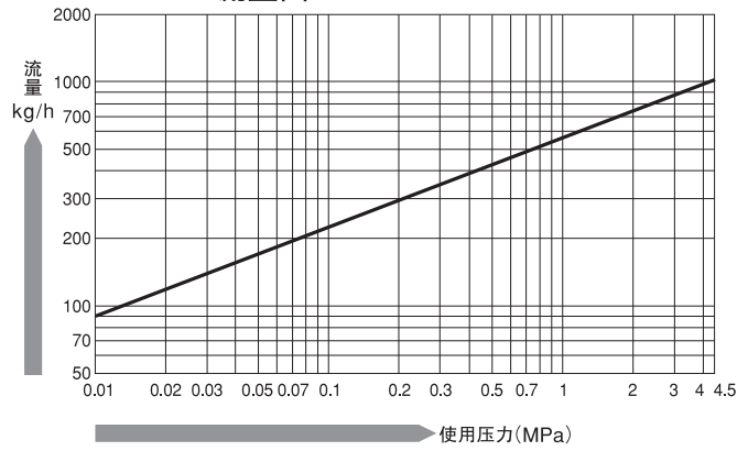
AGH12-流量图
